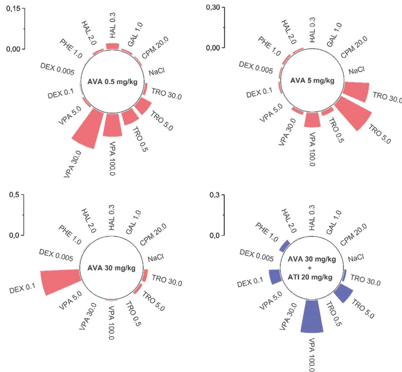
Рисунок 4. Радиальные диаграммы медианных значений вероятности сходства фармакологической активности аминоэфира вальпроевой кислоты (АВК, AVA) в дозах 0,5, 5 и 30 мг/кг, а также АВК с антагонистом \alpha_2 -адренорецепторов атипамезолом (АТИ) с препаратами обучающей выборки, полученных с использованием НБК.
